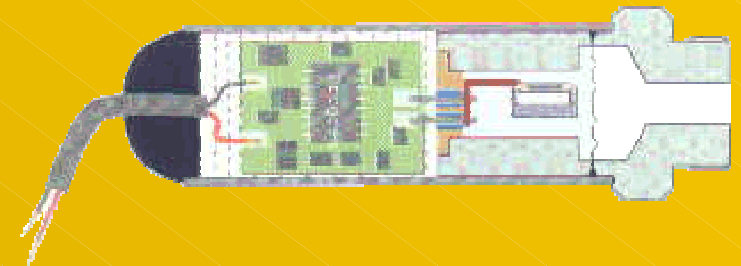
Transmissor de Pressão - montado
